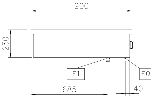
Zij aanzicht
