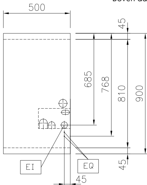
Boven aanzicht
